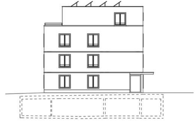
Ost-Fassade
